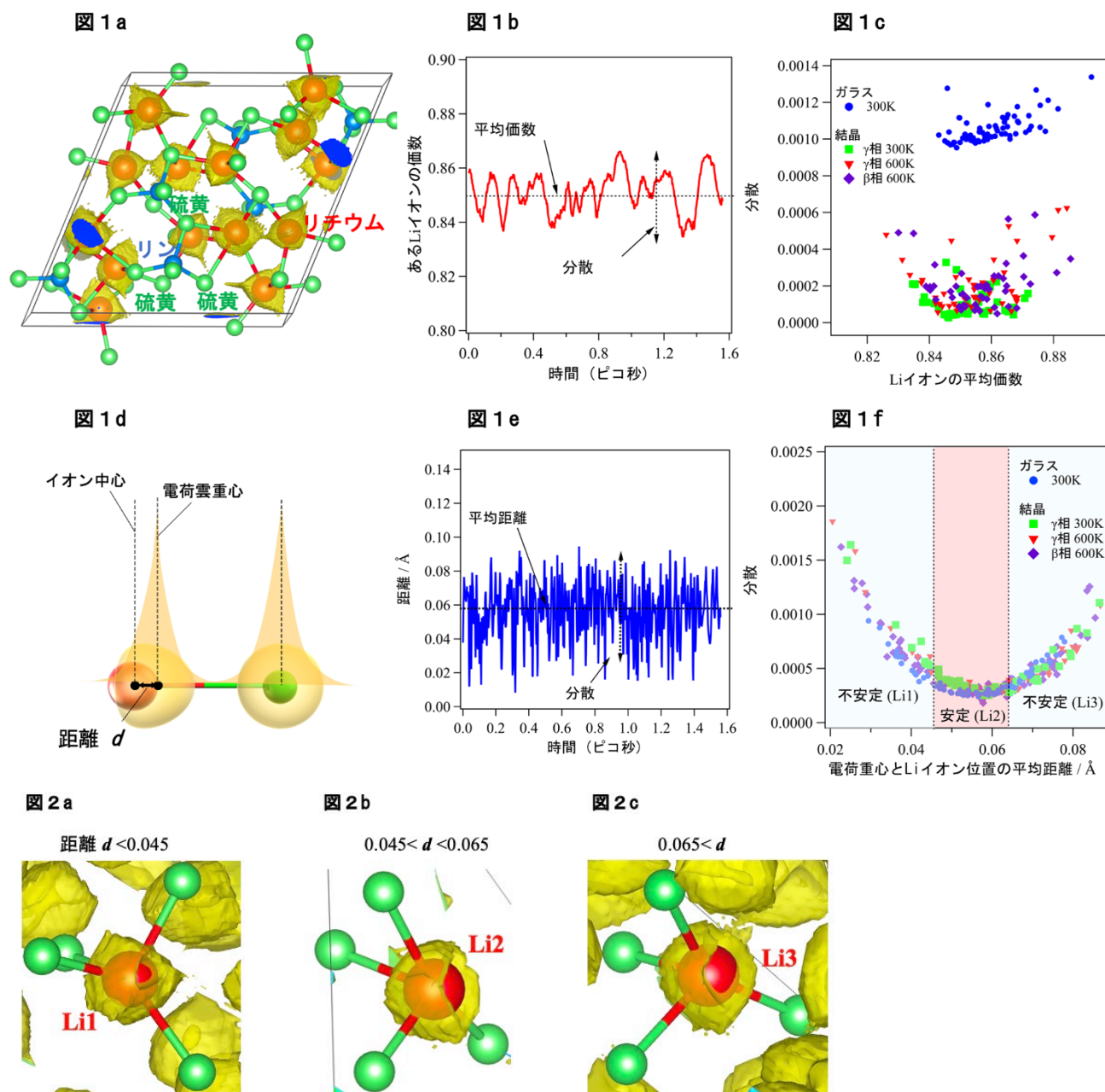
図1：Bader 電荷分析法で評価した Li イオンの環境。(a) \text{Li}_2\text{S}-\text{P}_2\text{S}_5 結晶の Bader 法から得られた Li イオンの電荷密度。(b) Li イオンの 1.6ps の間の平均価数振動と分散。(c) ガラス相 ※10 、結晶 \beta 相、結晶 \gamma 相の Li イオンの平均価数と分散の相関。(d) Bader 解析で得られる距離情報。(e) 1.6ps 間の Li イオン位置と電荷雲重心の平均距離と分散。(f) ガラス相、結晶相各々の Li イオン位置と電荷雲重心の平均距離と分散の相関関係。
